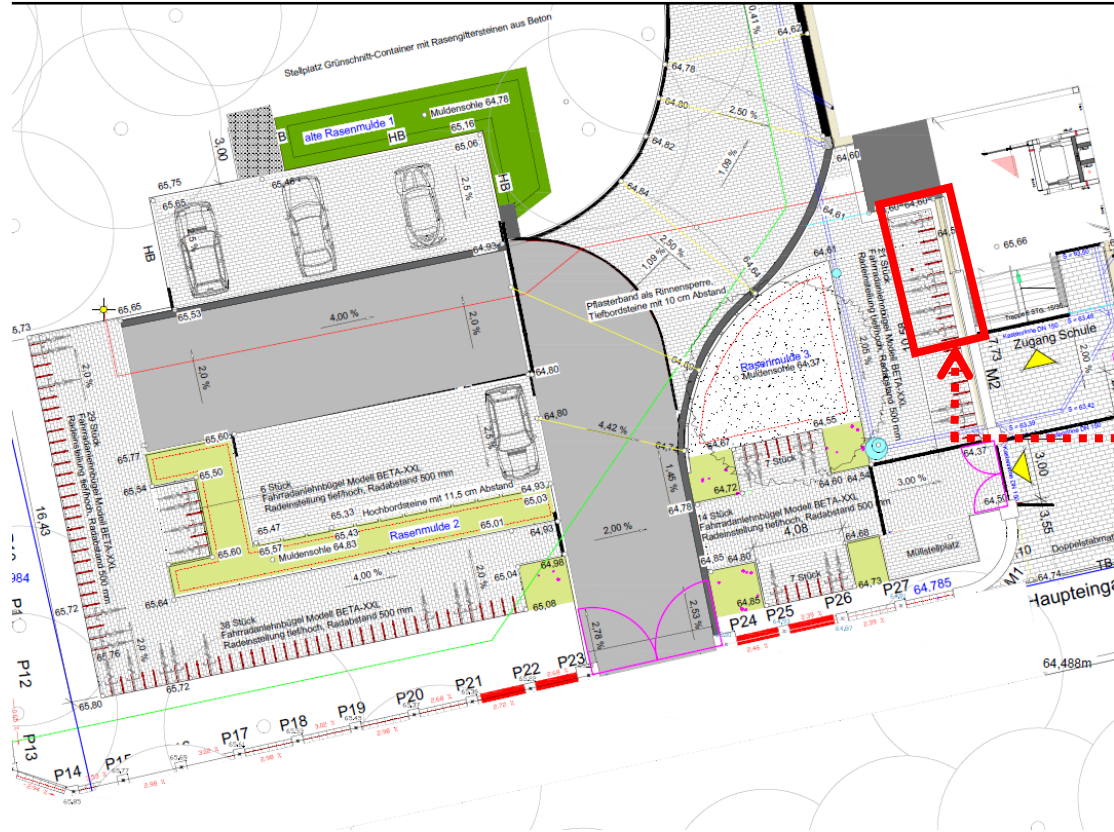
Auszug aus Plankonzept für ein neues Fahrradabstellsystem, Stand: 03/2025
