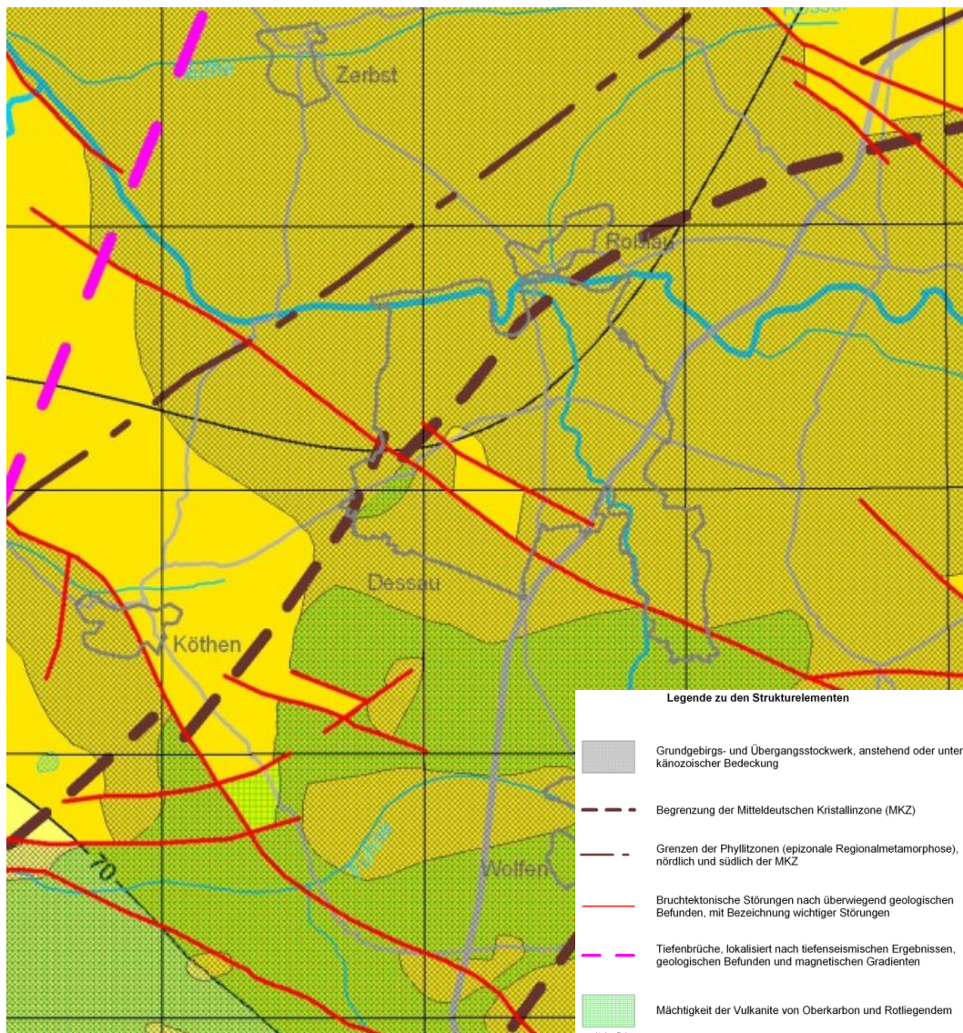
Abbildung 6-9 Ausschnitt aus der geothermischen Übersichtskarte von Sachsen-Anhalt mit geologischen Strukturen (Geothermische Übersichtskarte von Sachsen-Anhalt mit geologischen Strukturen, 1999)
