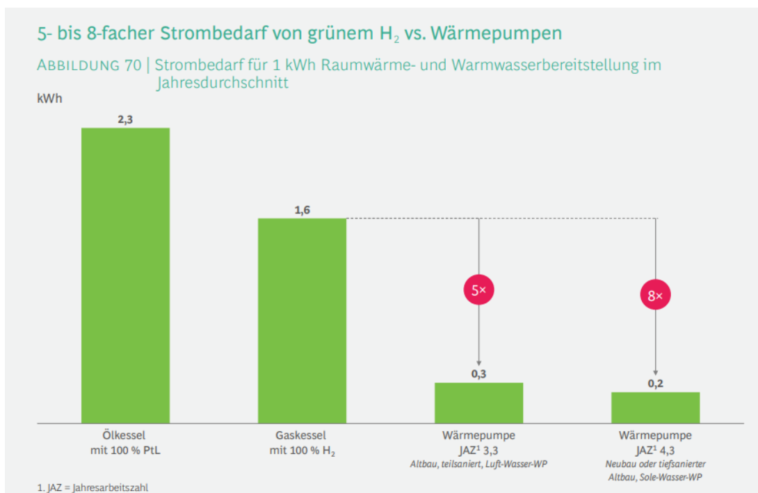
Abbildung 6-15 Strombedarf von verschiedenen Technologien zur Bereitstellung von 1 kWh Raumwärme und Trinkwarmwasser im Jahresdurchschnitt (BDI, 2021)
