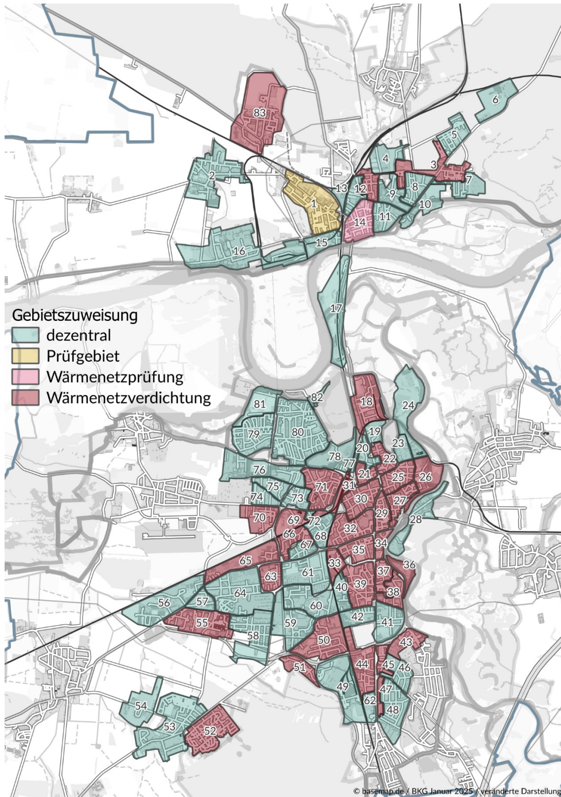
Abbildung 8-5 Eignungsgebiete für Fernwärme in der Stadt Dessau-Roßlau
