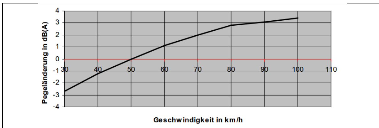
ABBILDUNG 13: Pegeländerung bei Änderung der Geschwindigkeit, bezogen auf 50 km/h (Beispiel: Landstraße mit DTV = 5.000 Kfz/24h)
