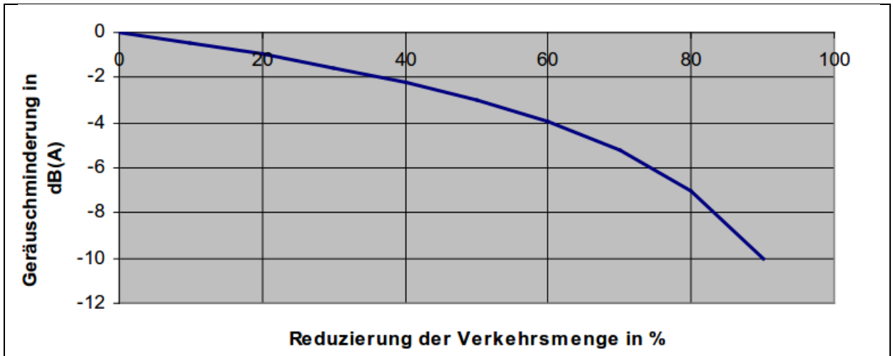
ABBILDUNG 11: Geräuschminderung durch Reduzierung der Verkehrsstärke
