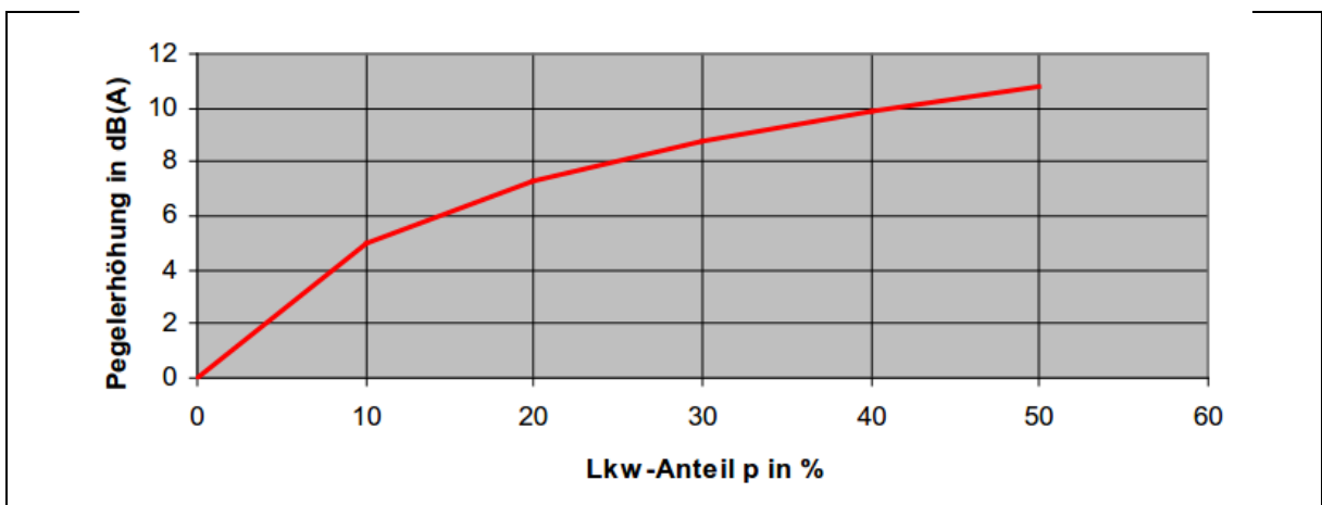
ABBILDUNG 12: Pegelerhöhung durch Erhöhung der Lkw-Anteile p (50 km/h)
