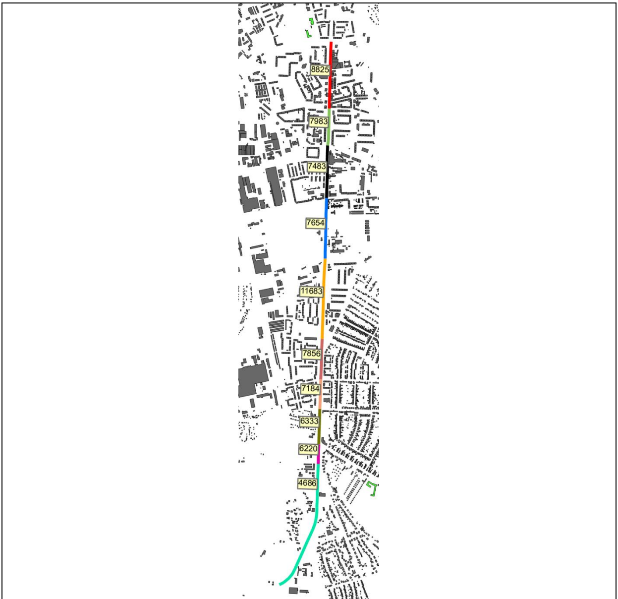
ABBILDUNG 4: „Straßenabschnitte“ der Heidestraße, gewählt auf Basis der DTV
